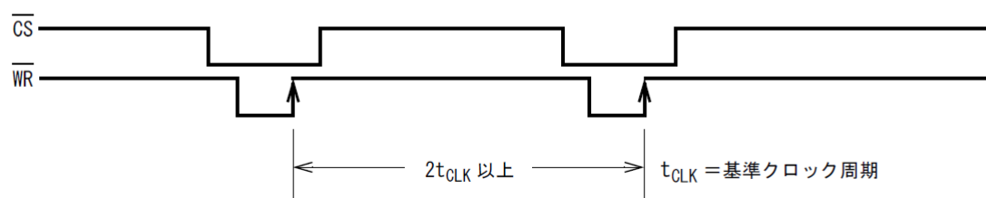
図 2-1:WRITE サイクルとリカバリタイム
